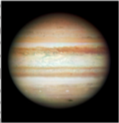
A La planète Jupiter
