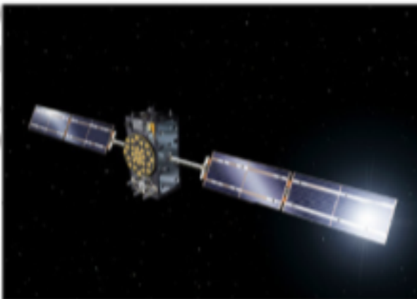
C Le satellite Galileo
